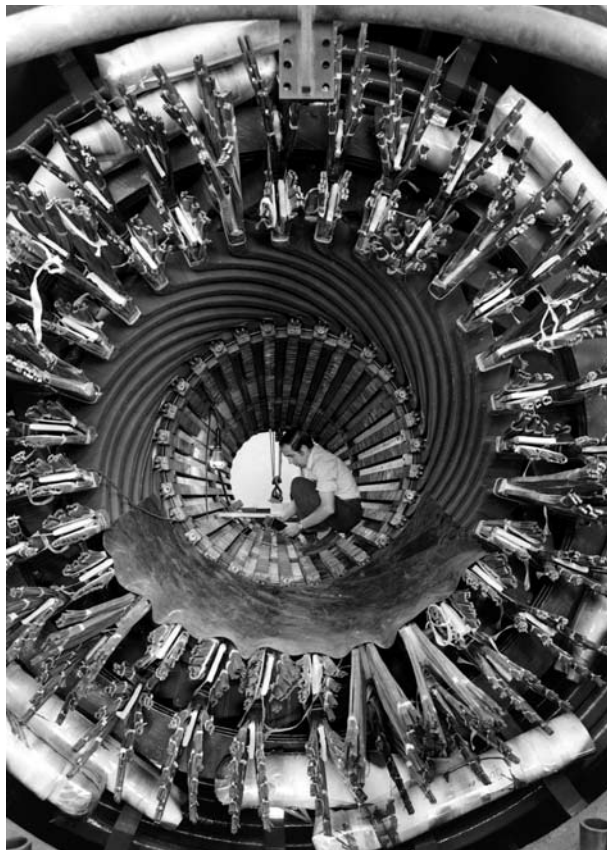
Fotografia industrial: Fàbrica Siemens, 1969
