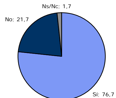
Fig. 2: Disposició d'intranet
