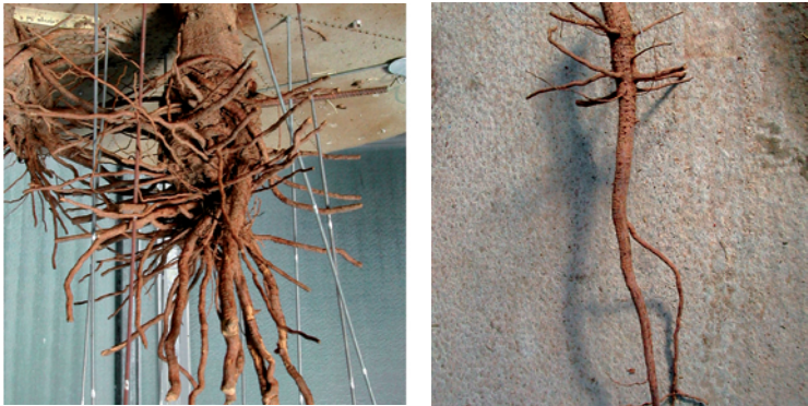
Fig. 4.4.1. Sistemas radicales adultos de pino. El superior muestra un crecimiento en espiral de las raíces como consecuencia del uso de bolsas de plástico en vivero. Ambos ejemplares proceden del vivero El Serranillo (DG Biodiversidad, MMA, Guadalajara).
