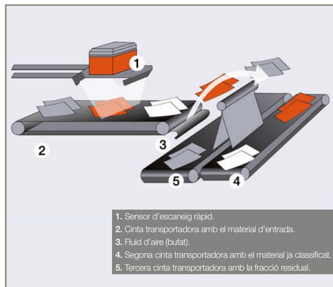
Figura 5: Components dels sistemes òptics.
